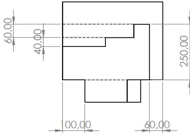
PLAN ASSISE BASSE
